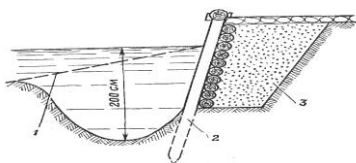
(Мал. 2) Укріплення берега палями:
